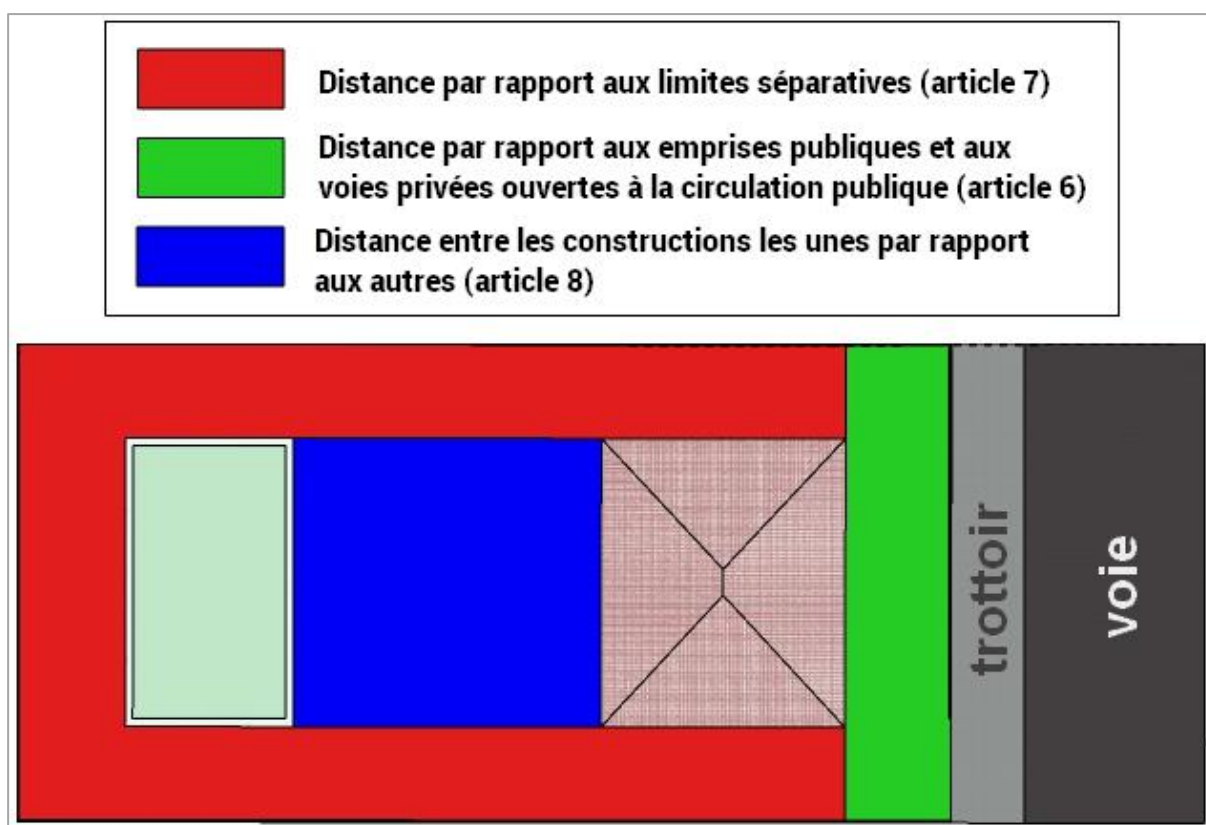
Règles d'implantation sur un terrain de 1000 m² comprenant deux maisons d'habitation
