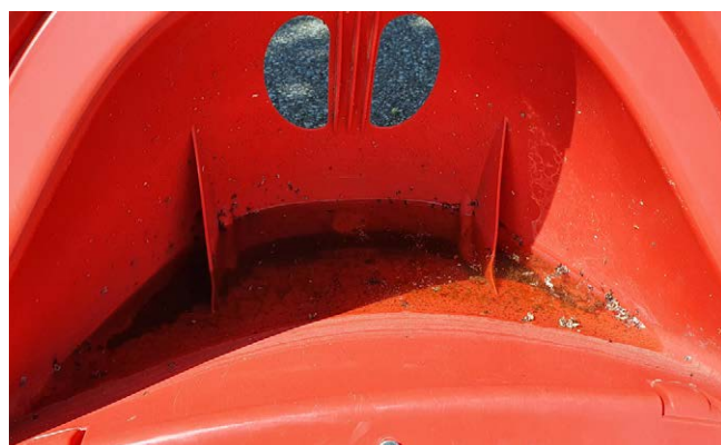
Exemples de lieux favorables à la présence de gîtes larvaires propices au développement du moustique-tigre
