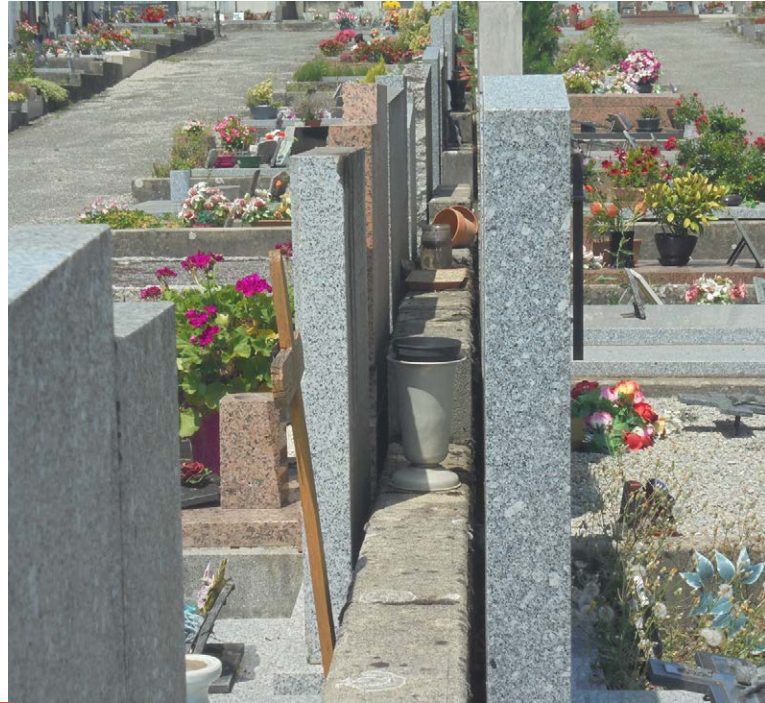
Exemples de gîtes larvaires propices au développement du moustique-tigre présents dans les cimetières
